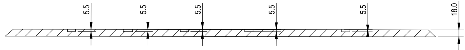
SECTION A-A SCALE 1 : 6
